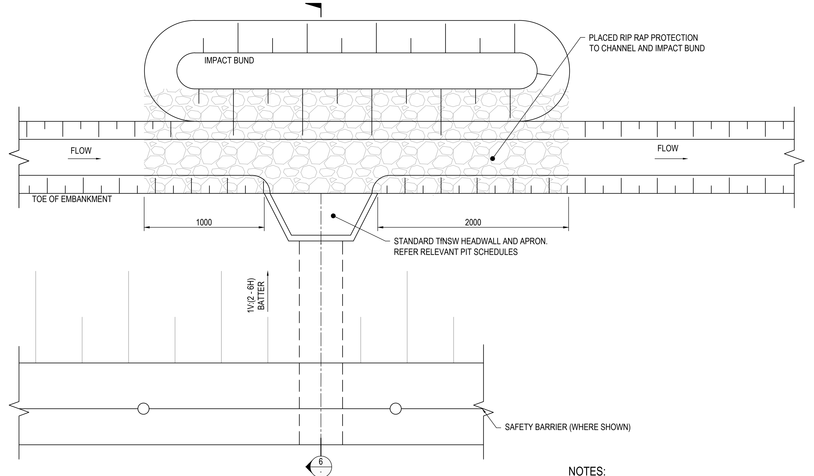
PIPE OUTLET TO CHANNEL SCALE: N.T.S
