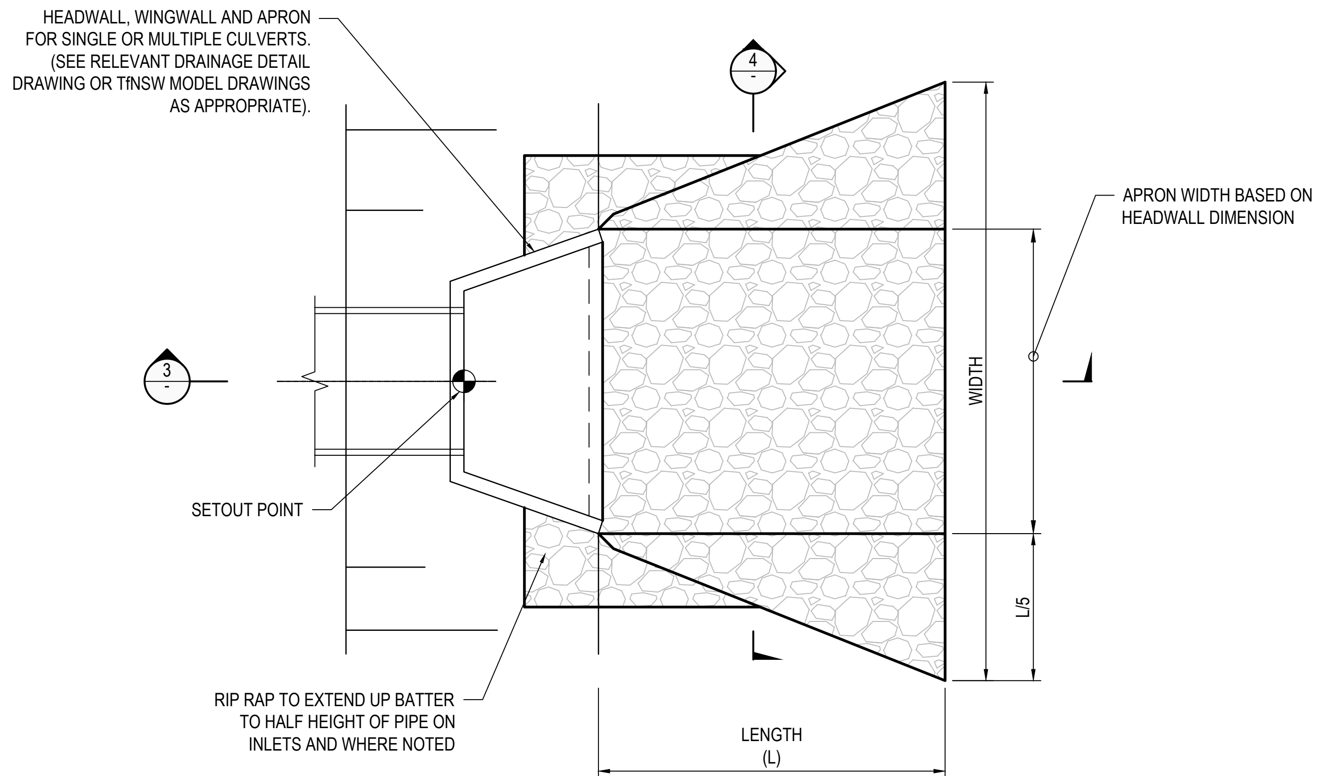
TYPICAL OUTLET DETAIL - RIP RAP SCOUR PAD SCALE: N.T.S
