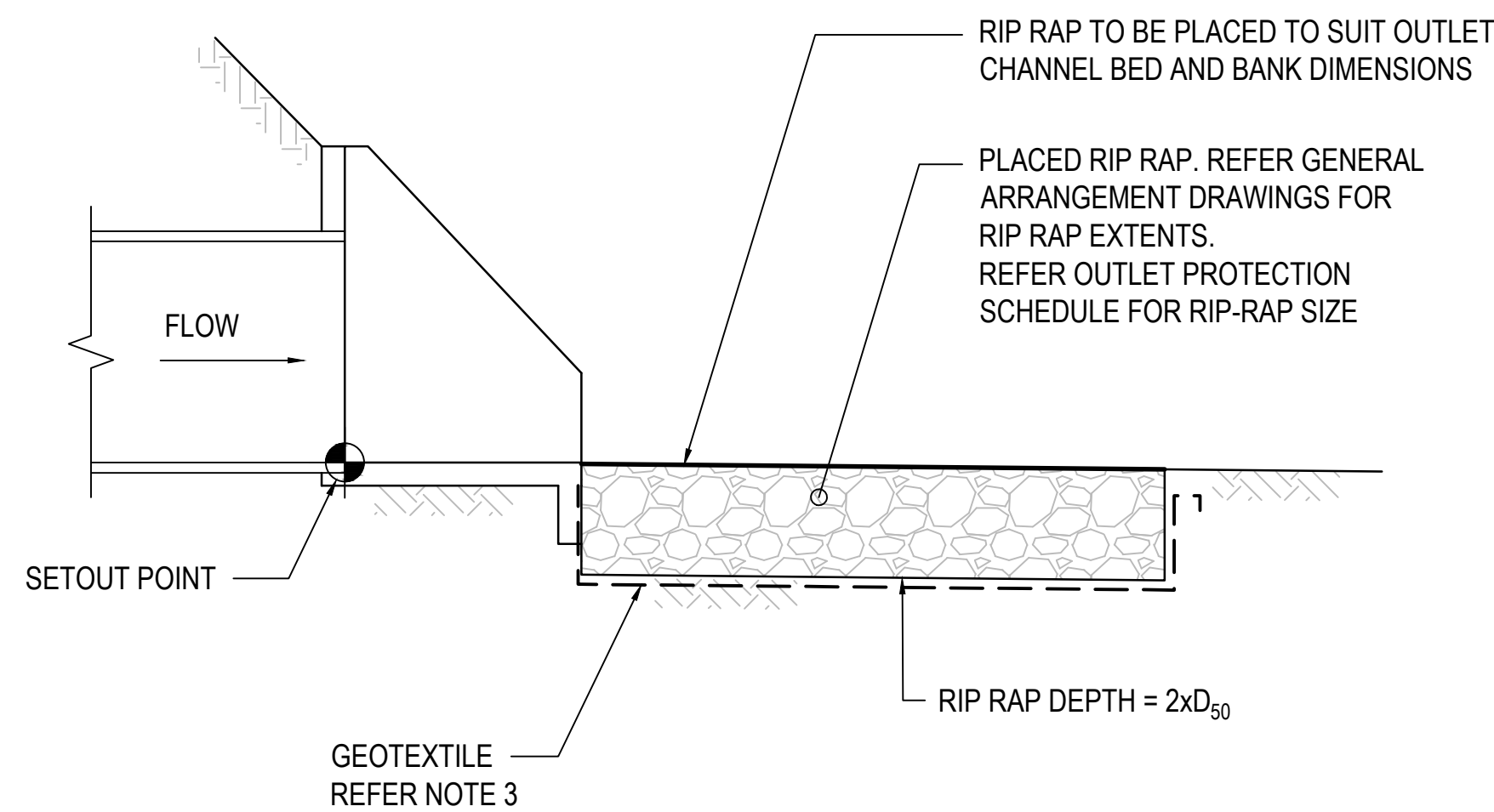
SECTION 3 SCALE: N.T.S
